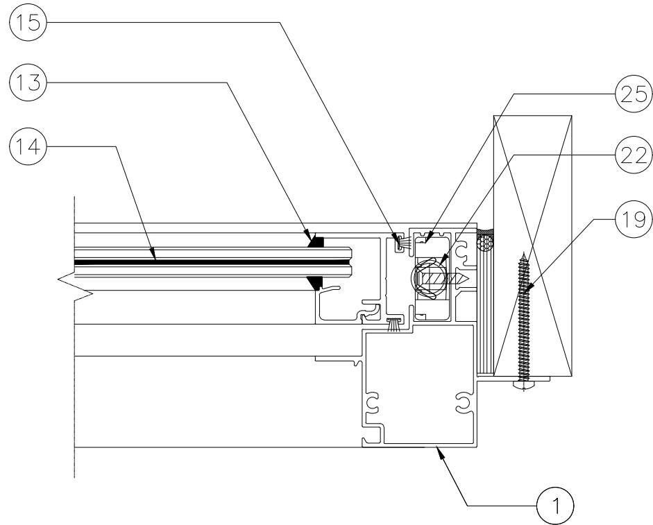
3 DETAIL D3
