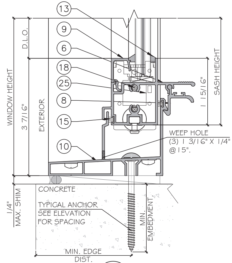
3 DI DETAIL
