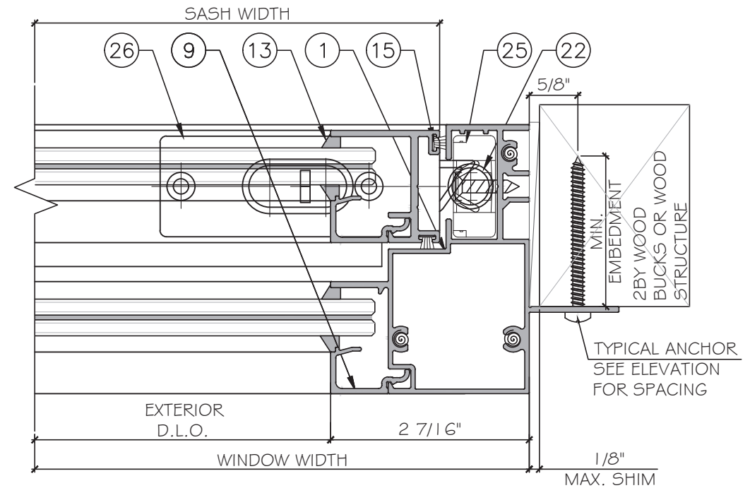
3 D3 DETAIL
