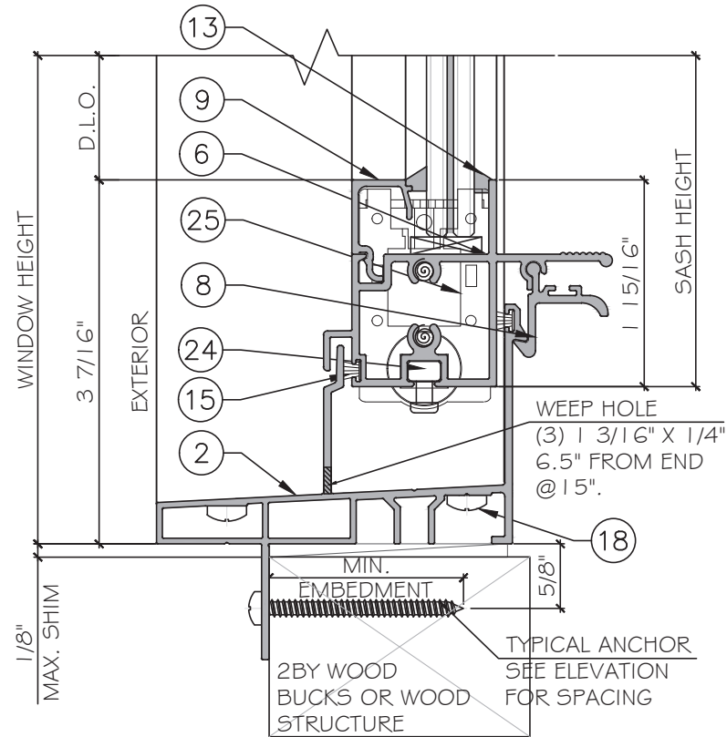
2 D3 DETAIL
