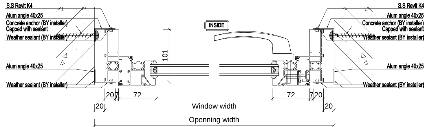
Section A-A
